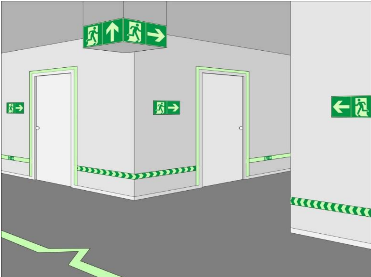
Рисунок А11 – пример комбинированного обозначения эвакуационного пути в широких коридорах, проходных помещениях и т.п. Тип ФЭС: G, Н
